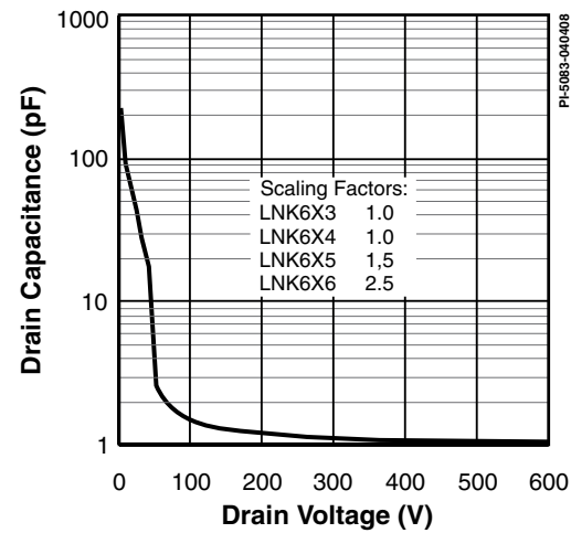
图 17. C_{OSS} 与漏极电压的特性曲线
