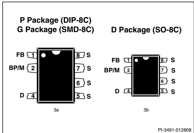
图 3. 引脚配置
