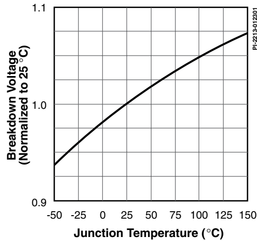
图 15. 关断与温度的特性曲线
