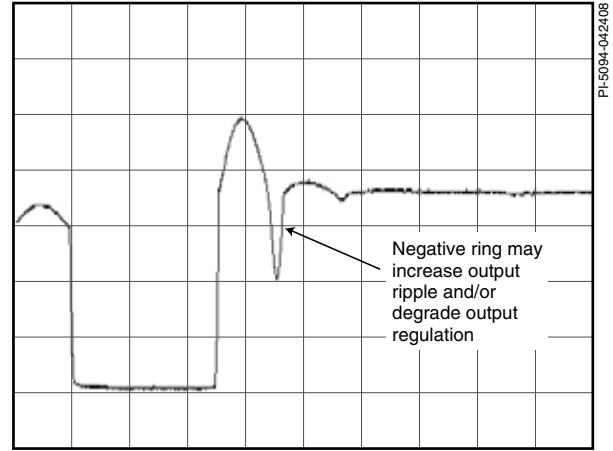
图 7. 具有大漏感振荡下冲的不理想的漏极电压波形
