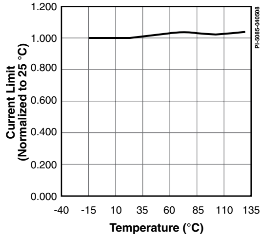
图 9. 电流限流点与温度的特性曲线
